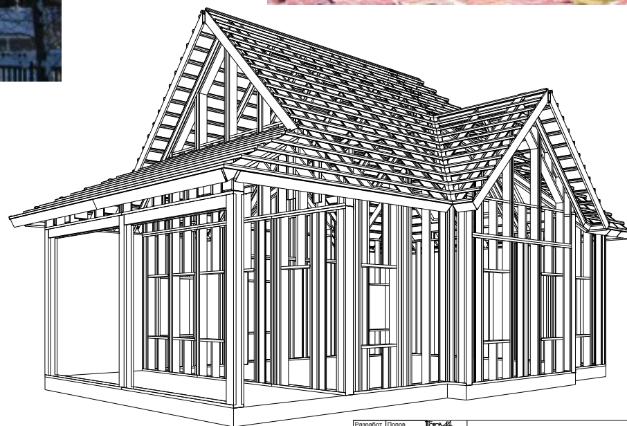
Проект жилого дома, 145 м2
